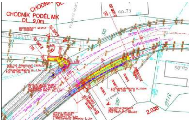
Situace řešení chodníku na konci obce
